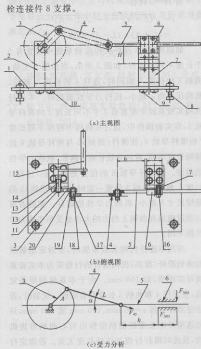
图1 连杆机构实验系统
