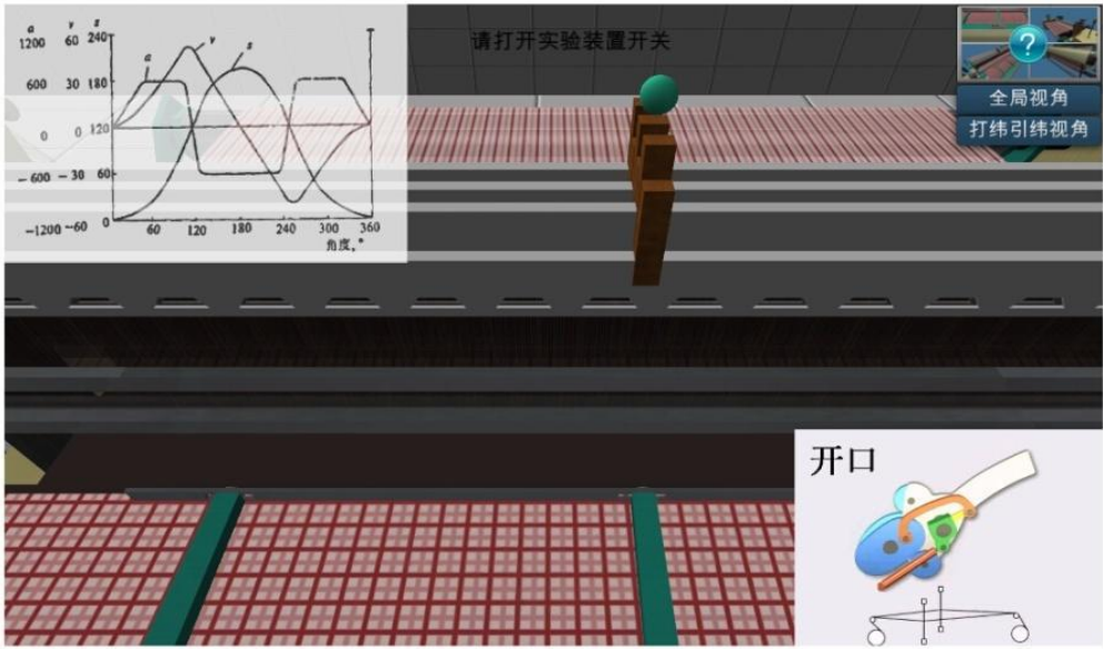
图2高速剑杆织机运动实验
