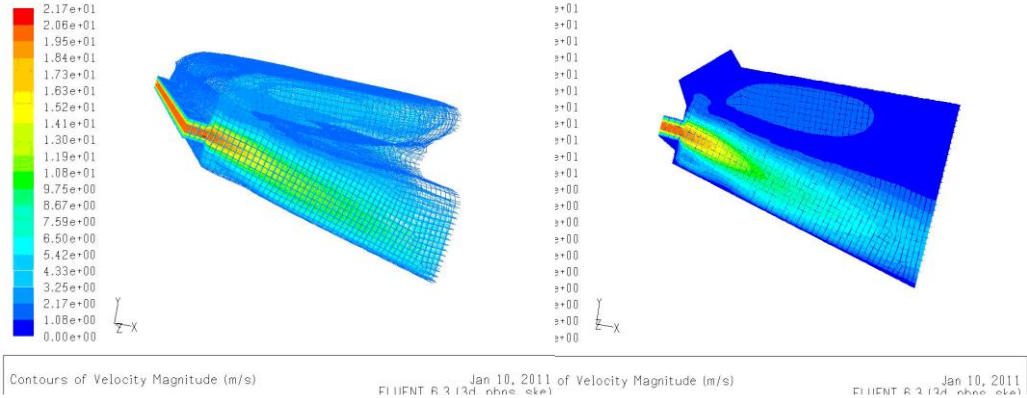
图3气流成网风道参数化虚拟设计实验
