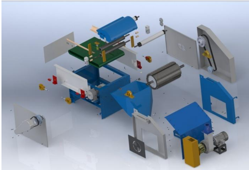
图4 松机整机装配虚拟仿真设计实验
